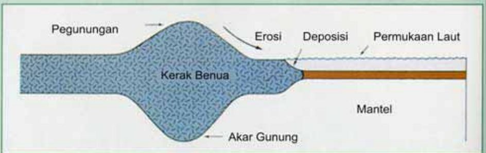
Ilustrasi lain yang menunjukkan bagaimana bentuk gunung menyerupai pasak, karena akarnya yang menghunjam dalam. ( Earth Science , Tarbuck and Lutgens, hlm. 158)
