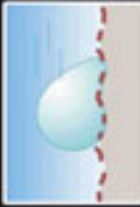
Su damlasının normal bir yüzeydeki etkisi
