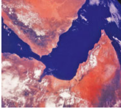
Yeryüzünün uydudan görünüşü.
