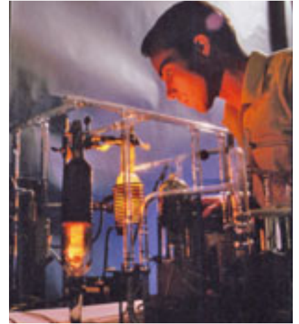
Kayaların yaşı, radyoaktif izlerin incelenmesi yoluyla da tespit edilir.
