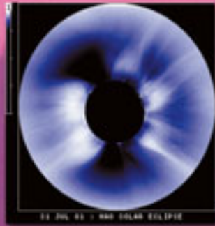
(Yukarıda) 31 Temmuz 1981 tarihinde gerçekleşen Güneş tutulmasının resmi.
